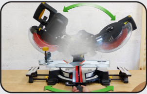
Tête inclinable gauche/droite Toutes commandes en face avant Double bevel All control panel in front
